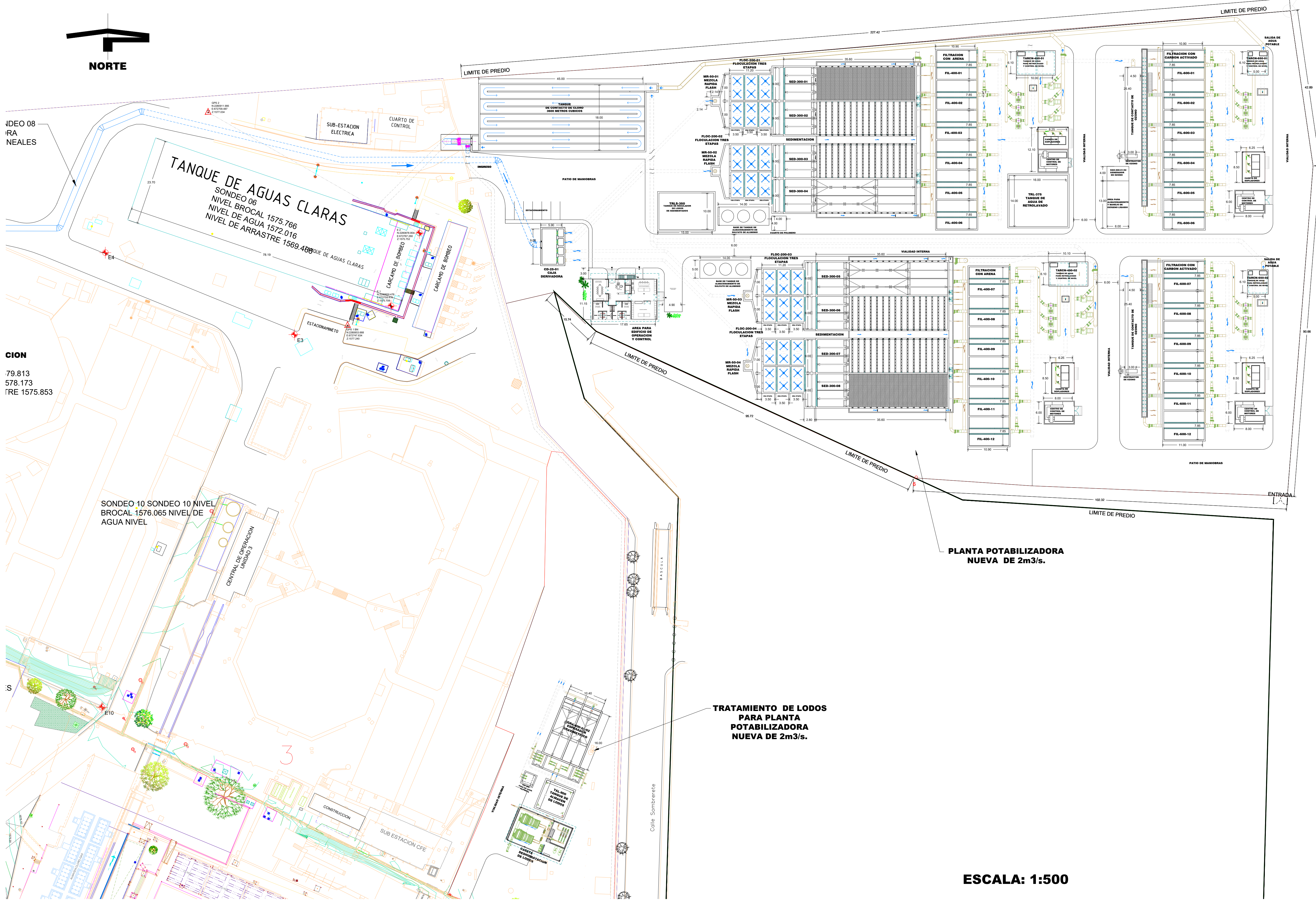
PLANO P02 A- ARREGLO GENERAL DE UNIDADES ESC:1:500
